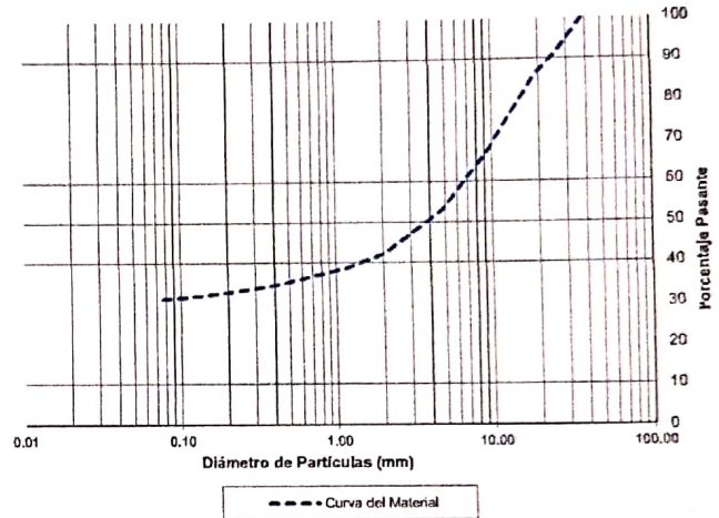
Curva Granulométrica
