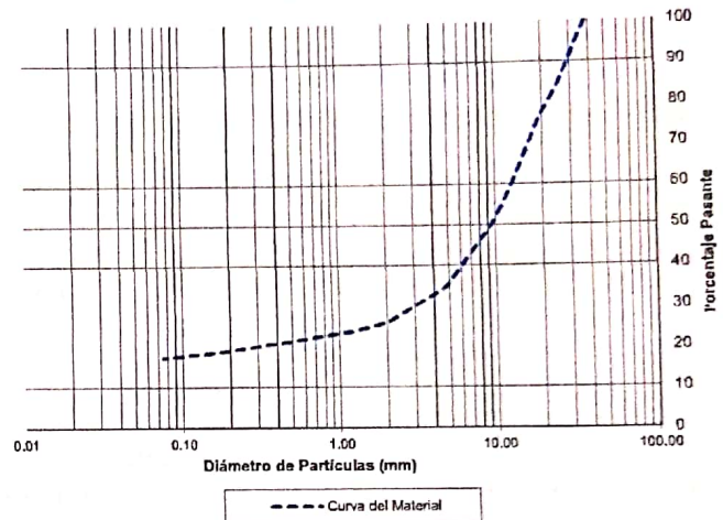
Curva Granulométrica
